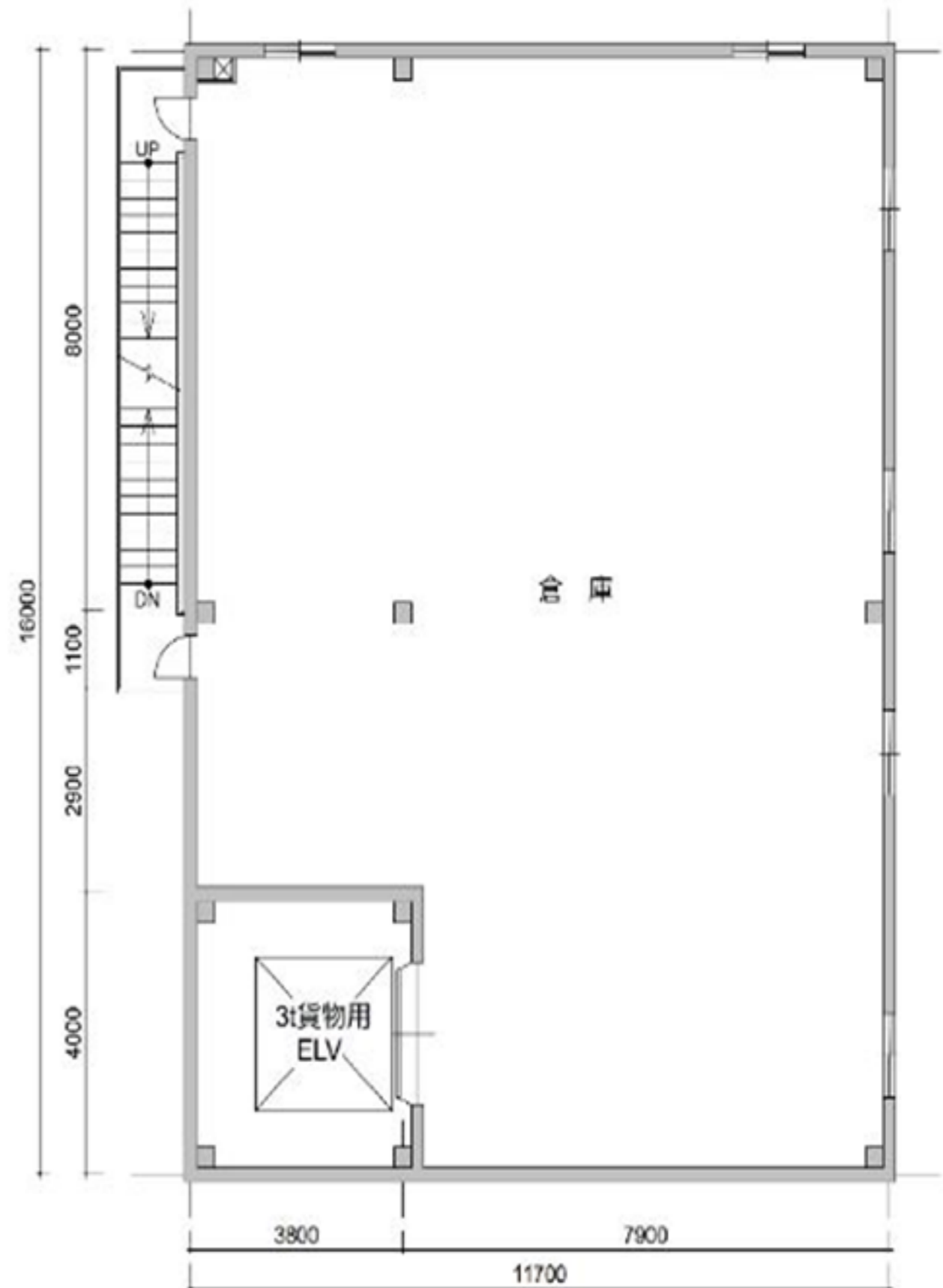
4階 平面図
