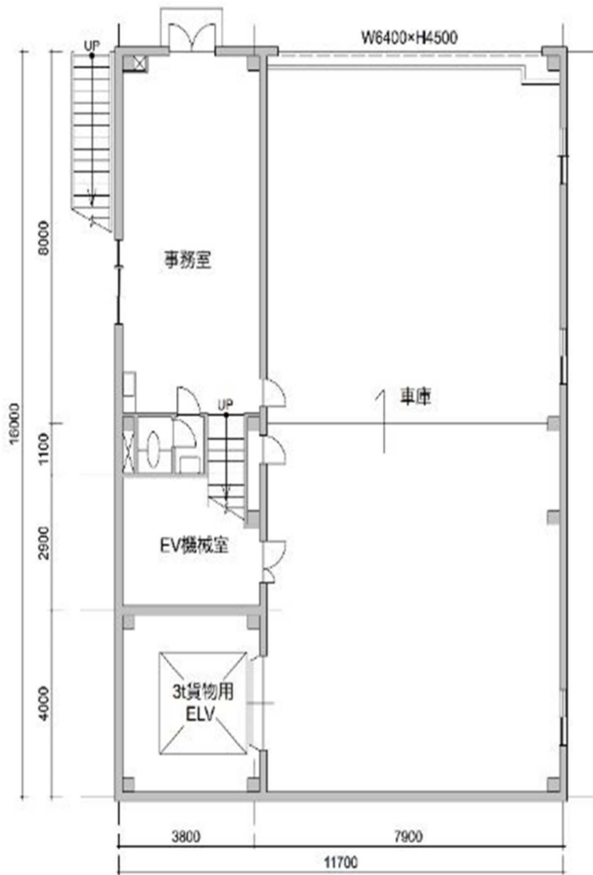
1階 平面図
